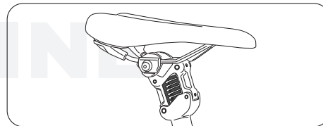
Fixation à la tige de selle suspendue
