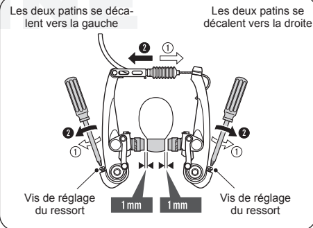
Réglage des freins au niveau de la jante
