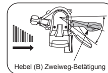
Hebel (B) Zweiweg-Betätigung Umschalten von einem großen auf einen kleineren Zahnkranz (Hebel B)
